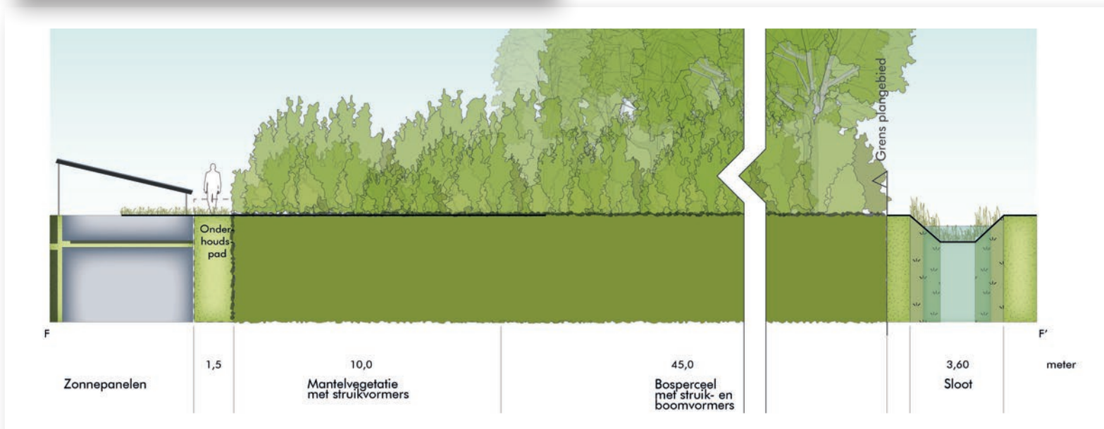
Doorsnedes E en F
