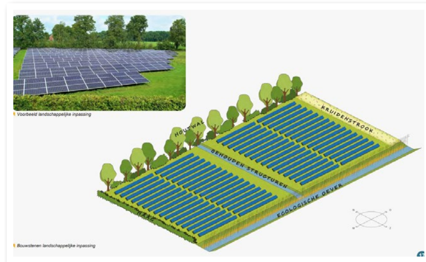
Bouwstenen voor een landschappelijk ingepast zonneveld in een open gebied
